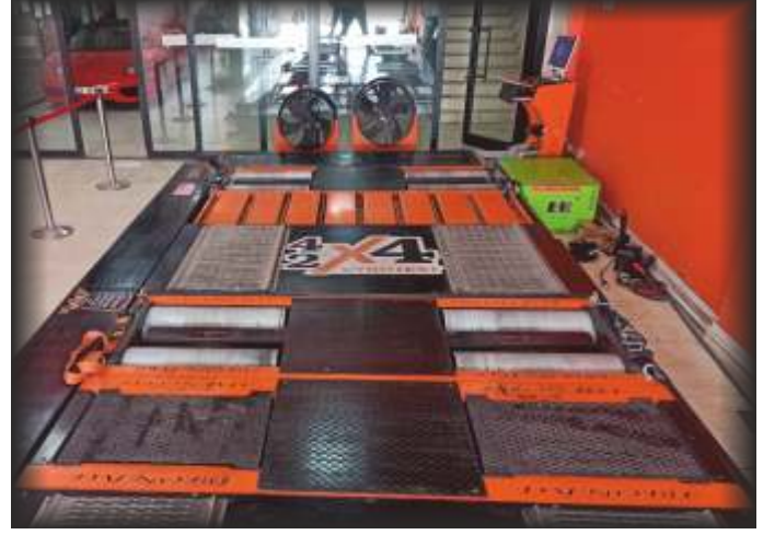
XR 1200 4 WD Senkronize Sistem + Manyetik Frenleme
